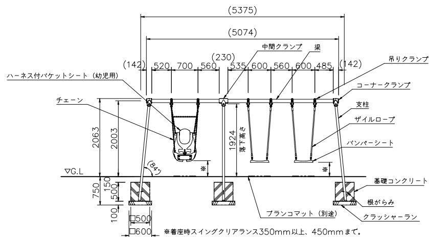
外観図 S=1/50
