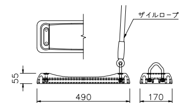
バンパーシート詳細図 S=1/10
