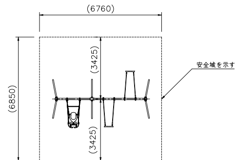
設置スペース 1/100
